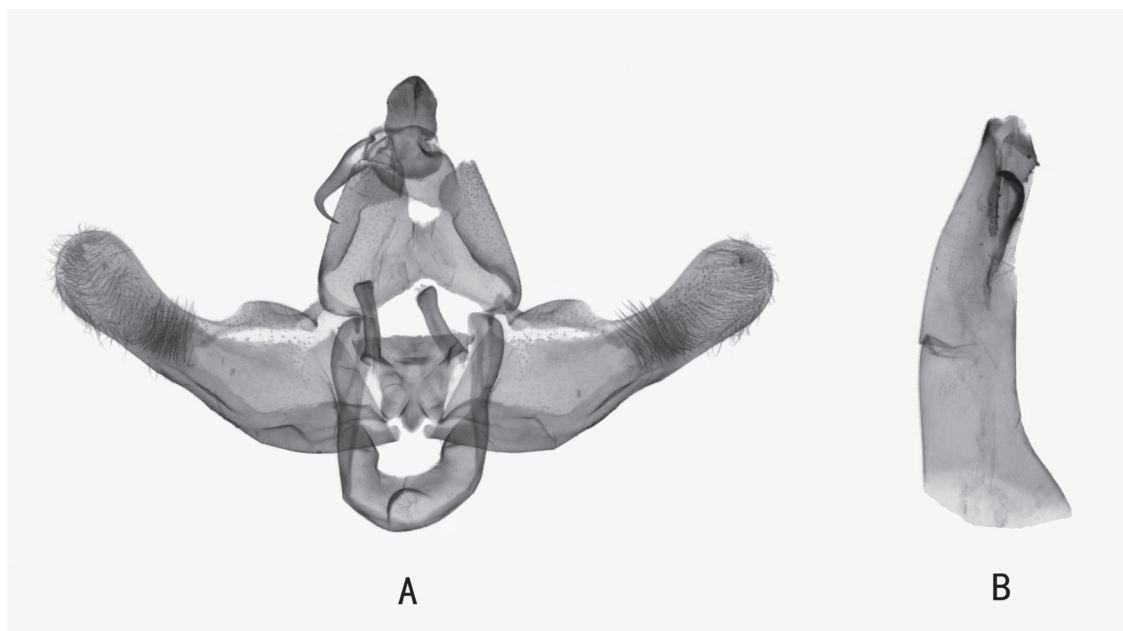
Fig. 5. Genitalia of Synersaga atriptera sp. nov. A. Genitalia. B. Aedeagus.
