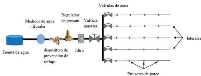
Figura 2. Esquema de un sistema de riego por goteo simplificado. Créditos: Haimanote K. Bayabil, UF/IFAS
