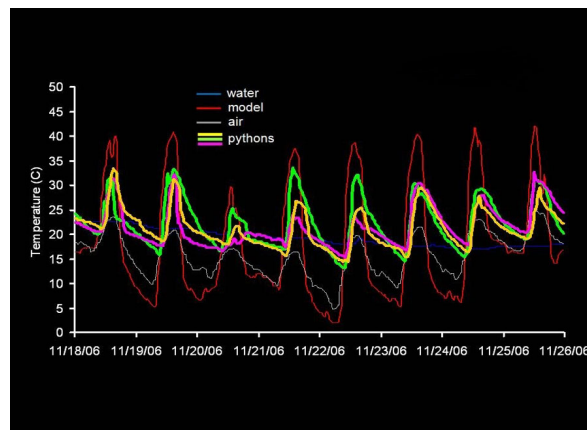
Fig. 5. Temperatura corporal de tres pitones Birmanas en el Everglades National Park, Noviembre 2006, mostrando las temperaturas predichas para los modelos biofísicos de culebras y las temperaturas del aire y del agua. Fuente: Davidson College.
